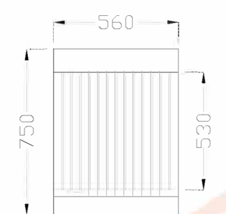
CA-56L ■瓦斯碳烤爐 560 x 750 x 300mm
