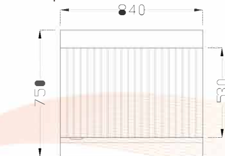
CA-84L ■瓦斯碳烤爐 840 x 750 x 300mm
