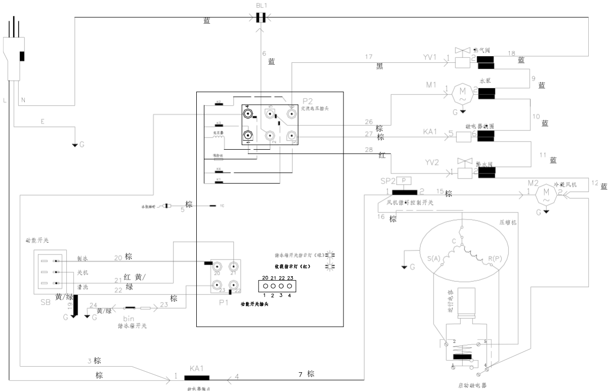
CM-105 接線圖
